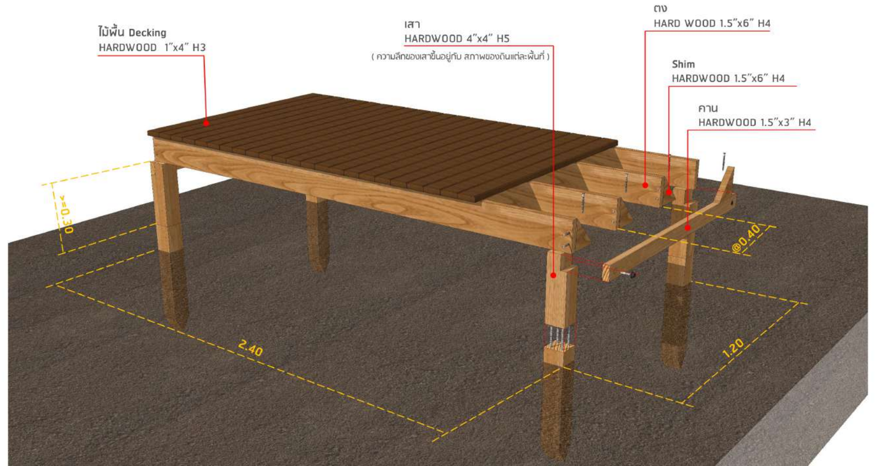
Decking Detail – 5 ( กรณีที่มีการต่อเสาเพิ่มความสูงของ Decking )
