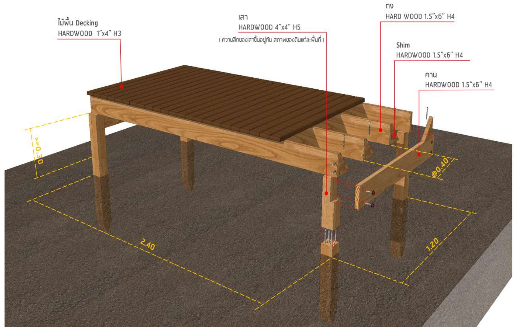
Decking Detail – 4 ( กรณีมีการต่อเสาเพิ่มความสูงของ Decking )
